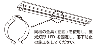
(図B) 落下防止金具
